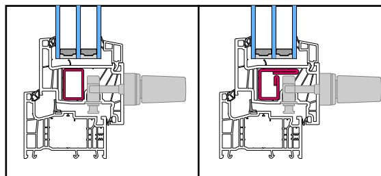
Nu sunt necesare prelucrări ale armăturii universale (stânga) și ale armăturii statice (dreapta).
