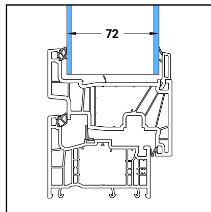
Canat coplanar
