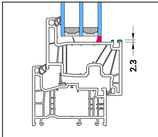
Soclu redus pentru baghetă pentru o lipire mai ușoară a geamului.
